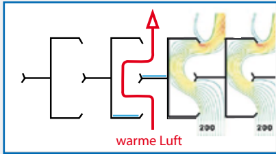
Ursprüngliche Geometrie Version 1 Cv= 0,296 des freien Querschnitts
