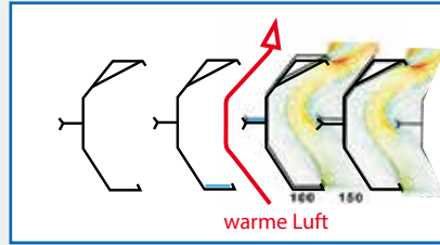
Ursprüngliche Geometrie Version 2 Cv= 0,414 des freien Querschnitts
