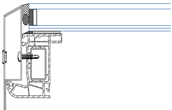
Die INDU LIGHT-Glasarchitektur-FLATLIGHT Konstruktion
